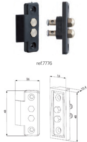
Contacto 2CN
