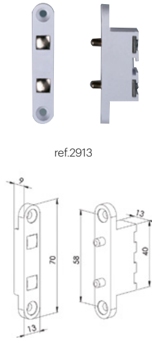
Contacto 2C
